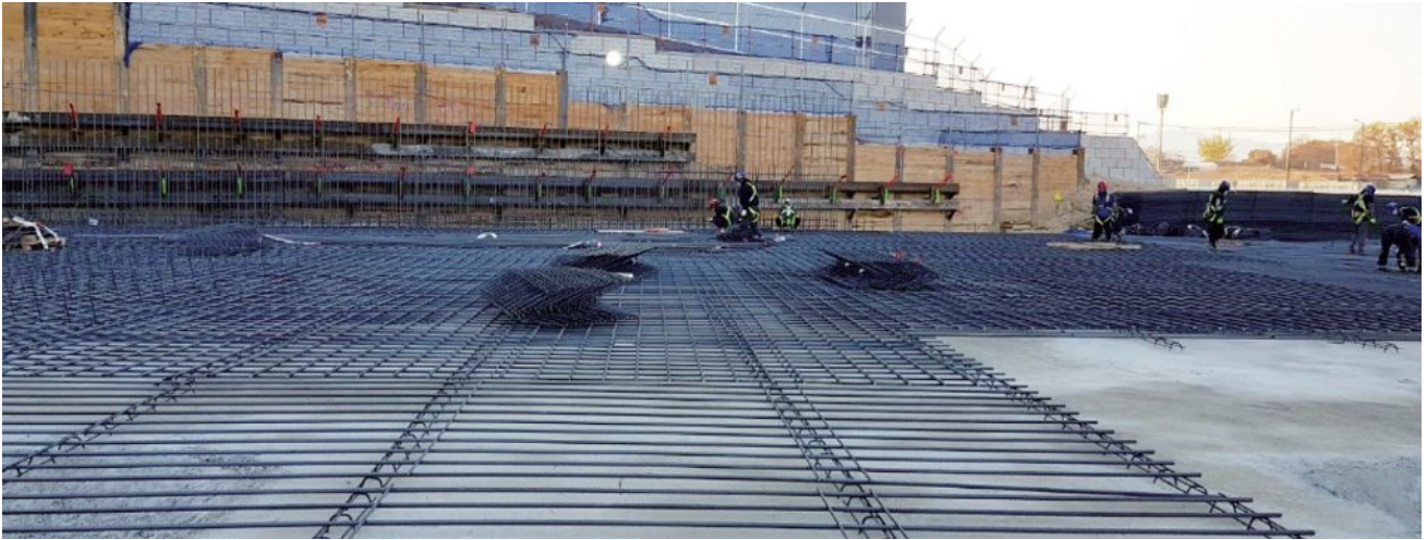
XY철근격자망 하부근 세로방향 설치
