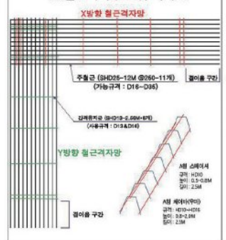
XY철근격자망 조립 사시도
