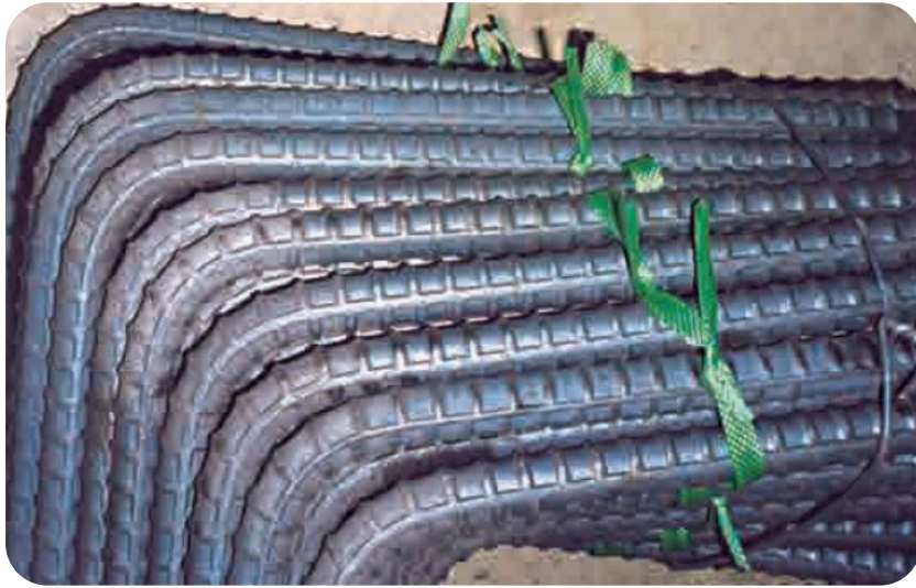
◎ 변화길이, 변화각 동시가공
